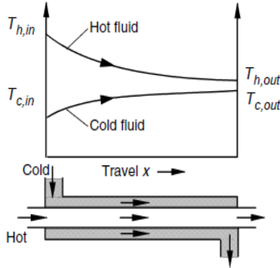
Şekil 4. Paralel aynı yönlü akış için sıcaklık eğrisi
